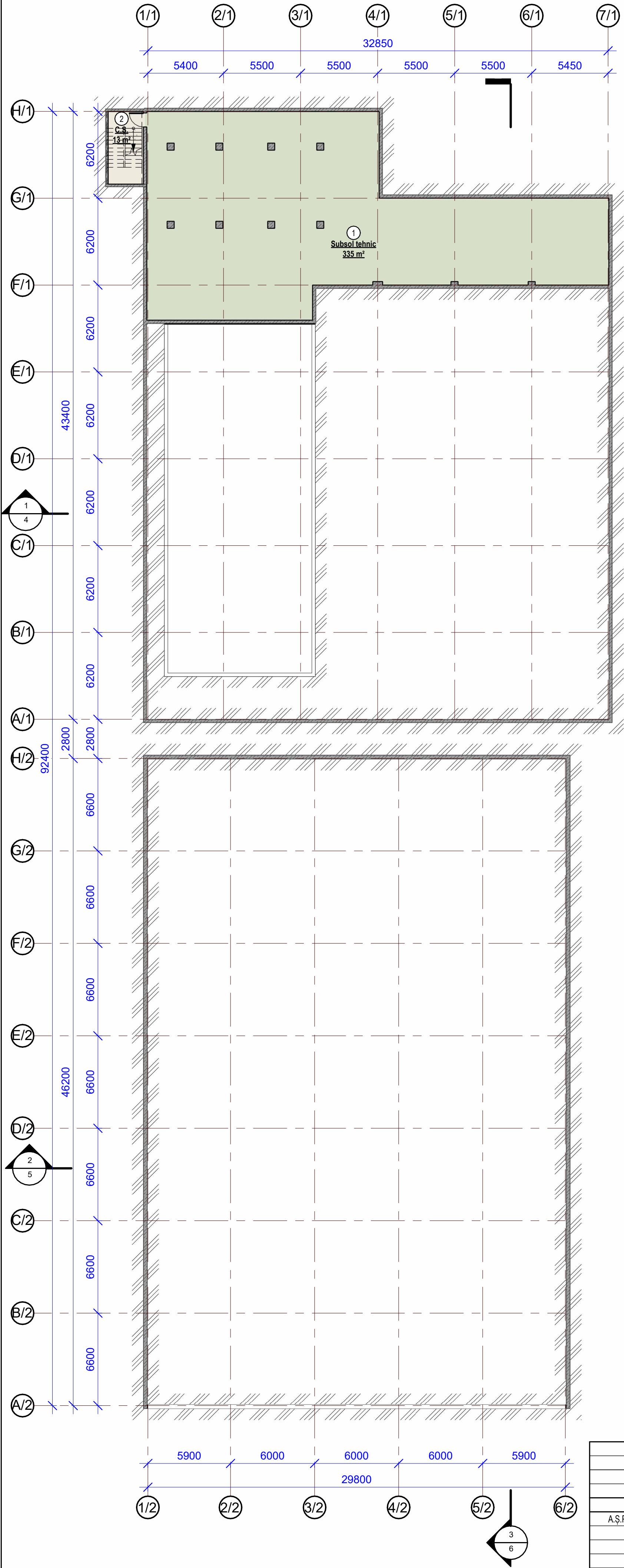
Plan subsol (cota -7.000), sc. 1:200
